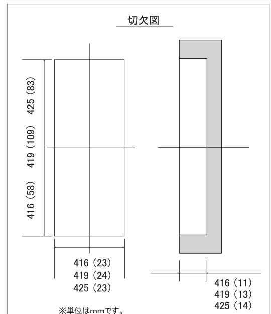
419取付図
