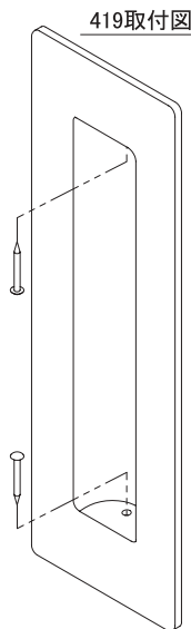
419取付図
