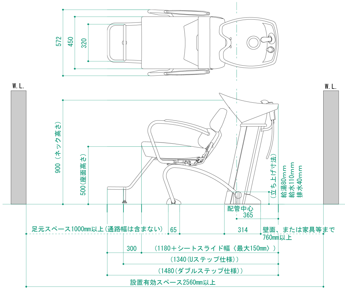
※ ( ) 内寸法は参考寸法。(図はSU-KFPLW/EX-NRS1)
