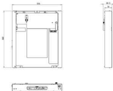
寸法図
