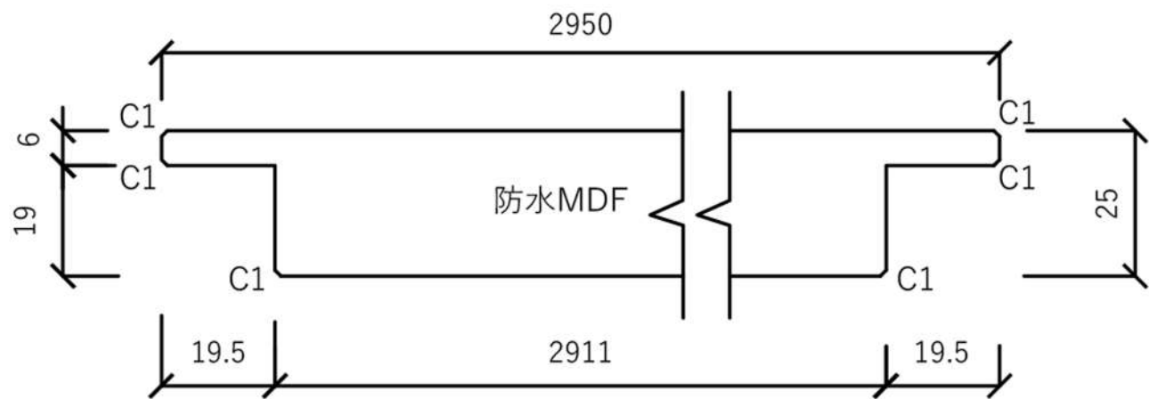
長手断面図
