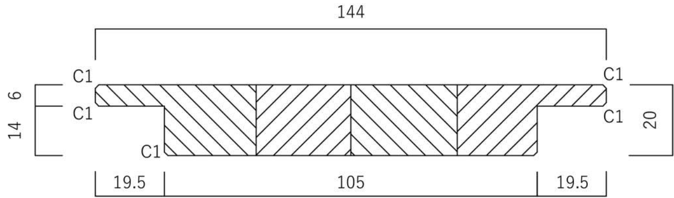
短手断面図
