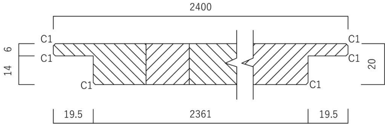
長手断面図
