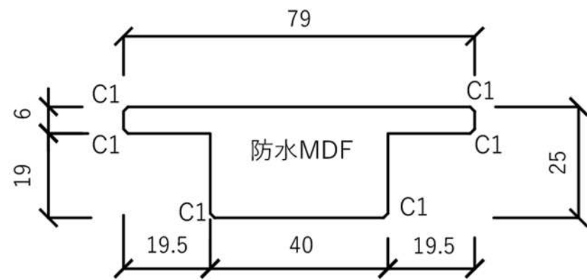
短手断面図
