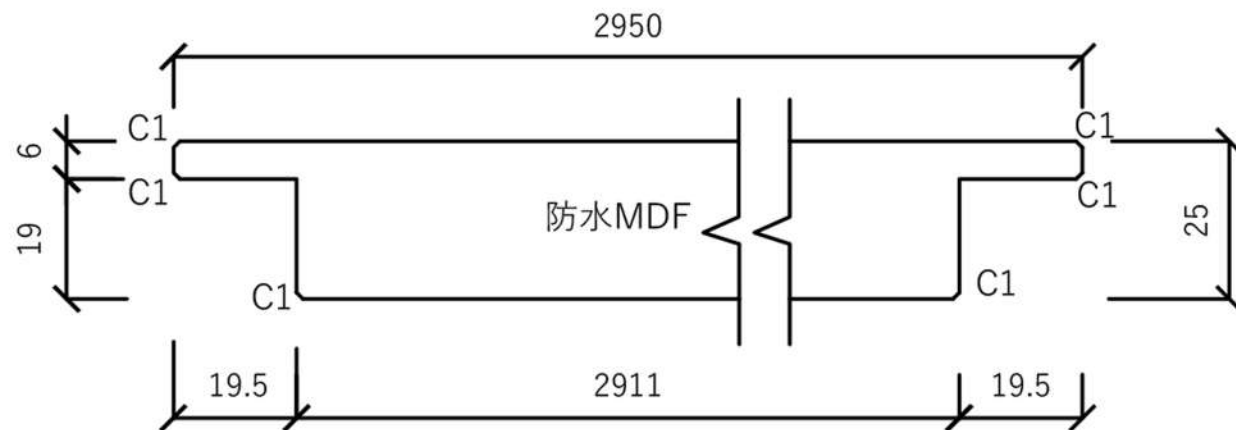
長手断面図
