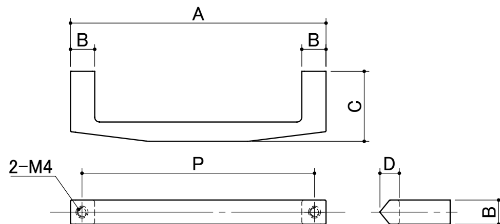
■ GRAVINE 寸法表
